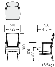
BR ¥ 52,500 張材：背：ビニールレザー【ランク外 (L-8197)】 座：ビニールレザー【ランク外 (L-8203)】
