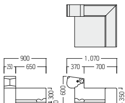
●S・OC-300・OF・KSC・H 角コーナー ヒツジ ¥ 160,000 張材：ビニールレザー [AL-10R/Q/D/H/36]
