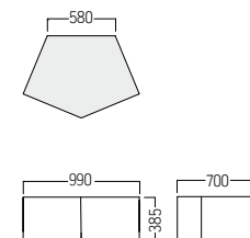
(固定式 23kg) (可動式 23.5kg)
