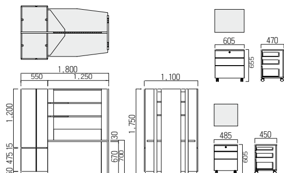
S·KJ-061・C 座頭台ロータイプ カギ付・前輪ストッパー付キャスター
