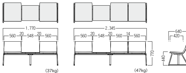
充電タイプ 中間脚からケーブルが出ています。
