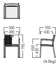
●S・CG-326・B ㊦ ¥55,700 主材：アルミパイプ・ポリエチレン編み 肘：木目調ポリエチレン
