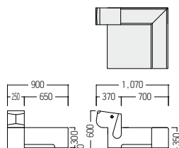
●S・OC-300・OF・KSC・I 角コーナー イヌ ¥ 160,000 張材：ビニールレザー [AL-10R/H/36]
